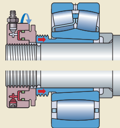
Стяжная втулка
