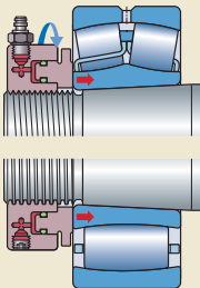
Конический вал
