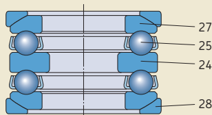
Двойной упорный шарикоподшипник
