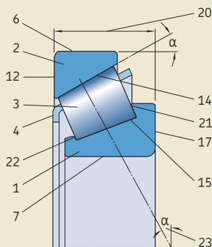
Конический роликоподшипник
