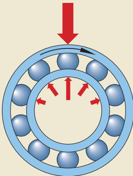
Распределение нагрузки
