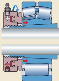
Закрепительная втулка
