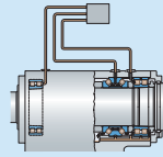
Масловоздушное смазывание
