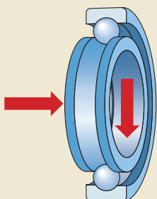
Распределение нагрузки
